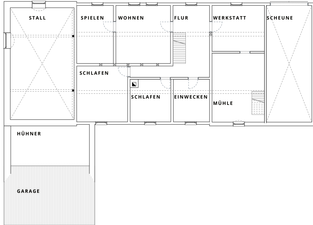
Obergeschoss Bestand
