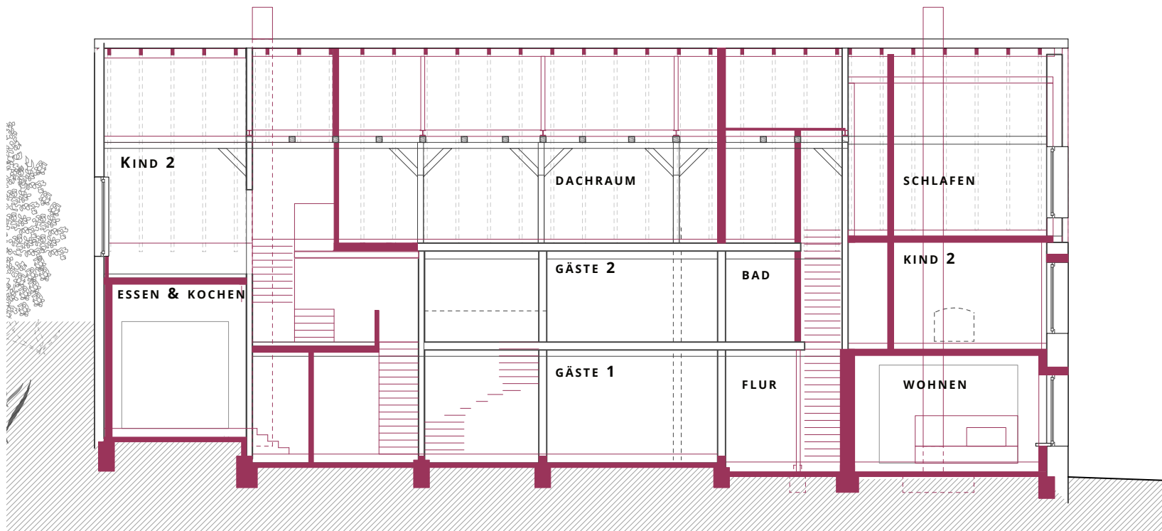
Längsschnitt Neu
