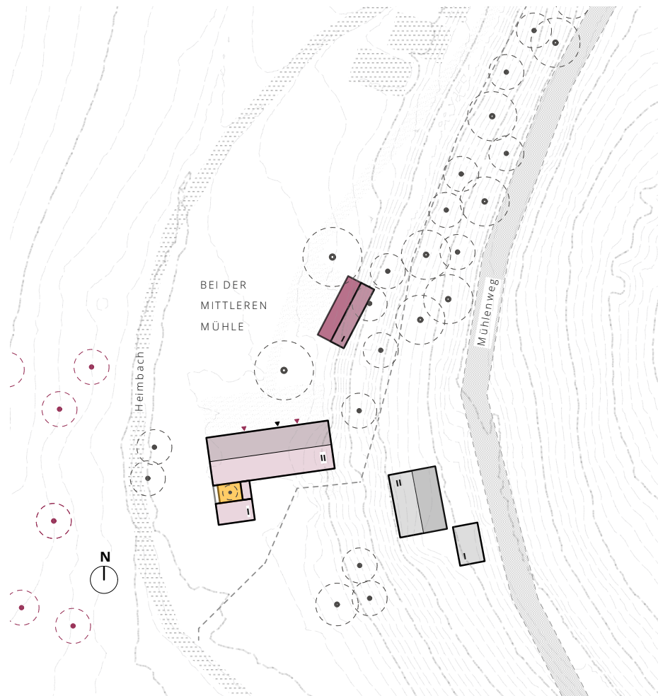
Lageplan
