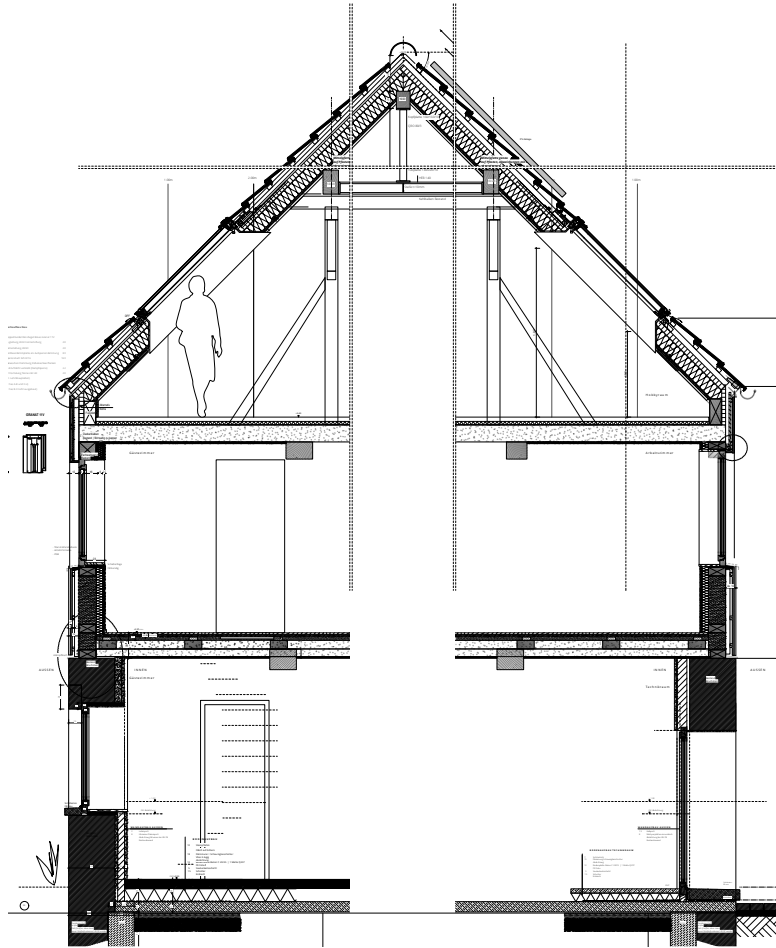
Detailschnitt B-B
