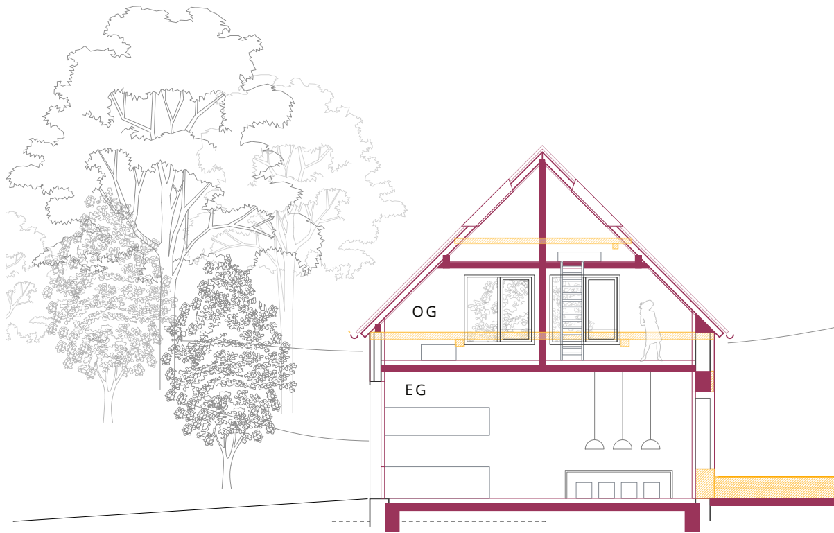
Schnitt A-A
