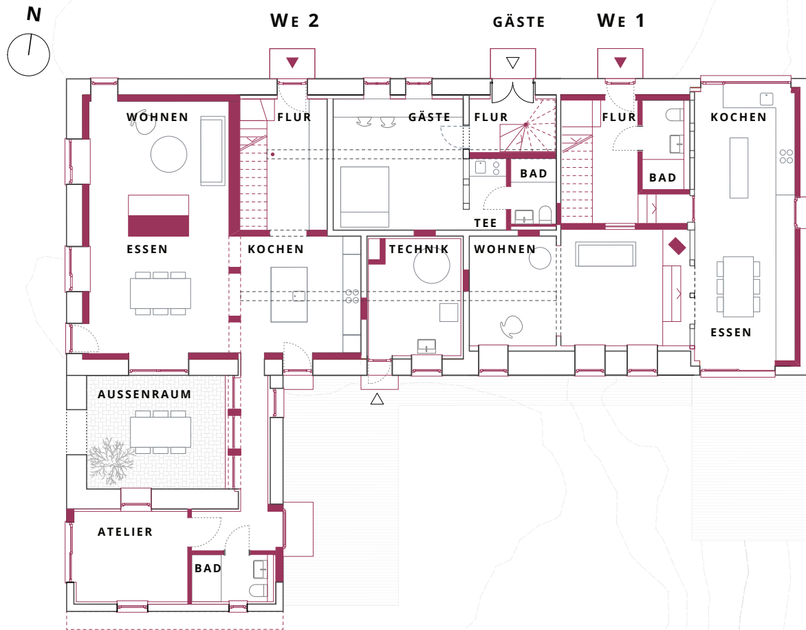
Erdgeschoss Neu
