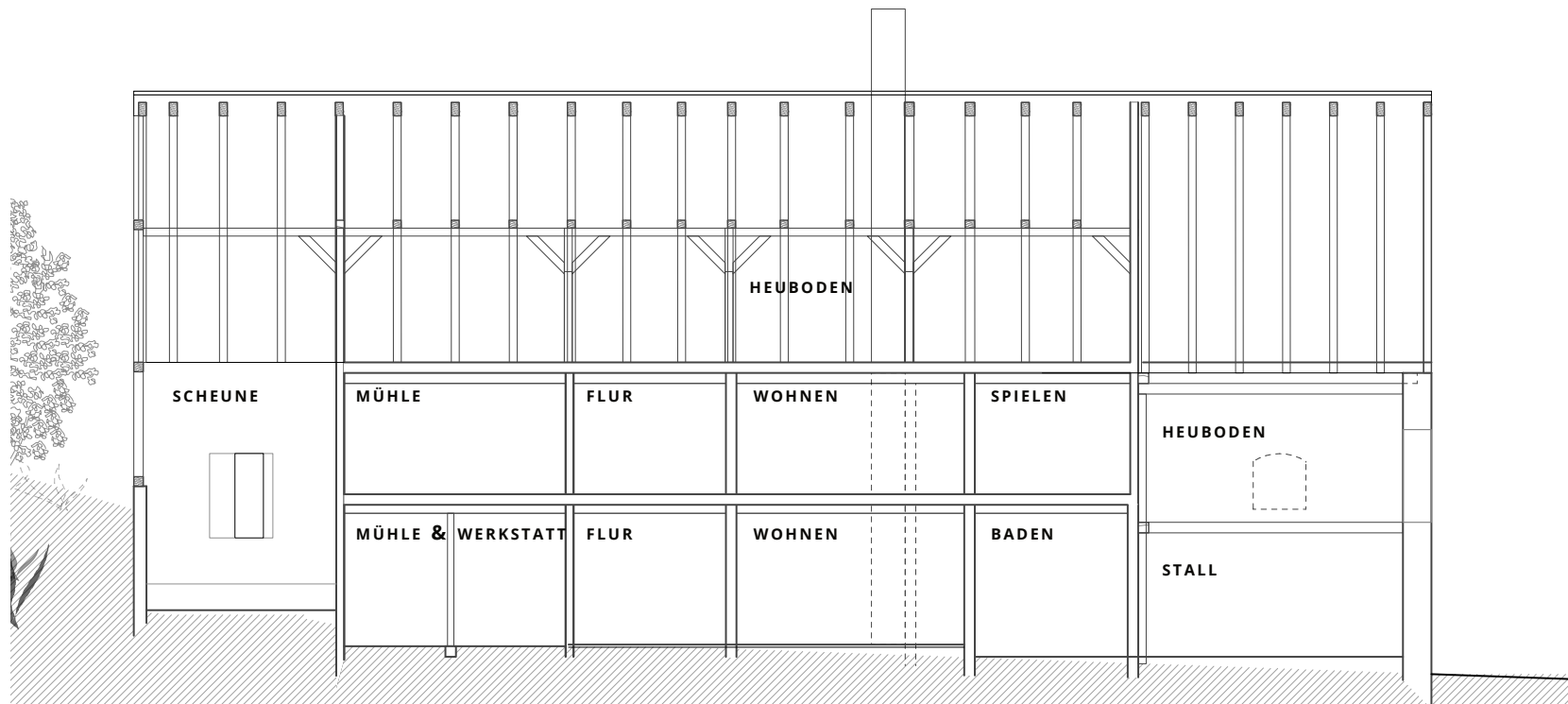
Längsschnitt Bestand
