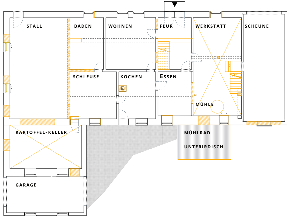
Erdgeschoss Abbruch
