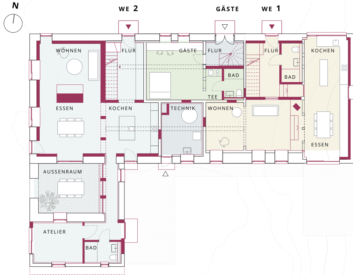
Erdgeschoss Neu Wohneinheiten
