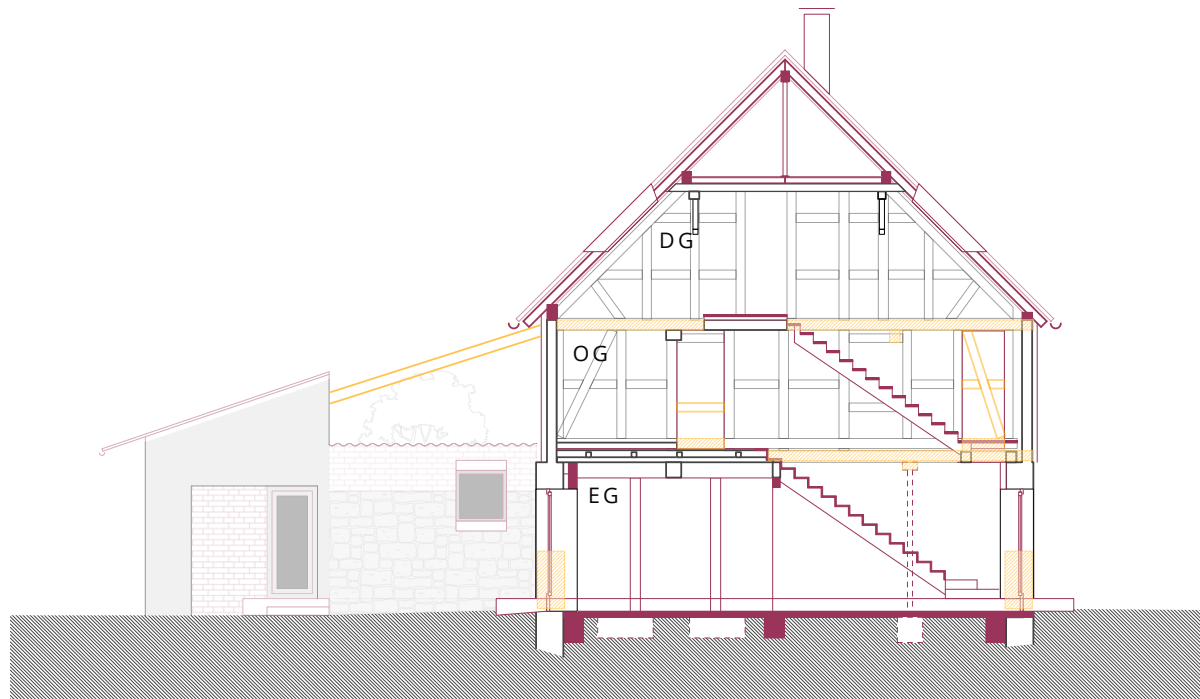
Schnitt-Ansicht
